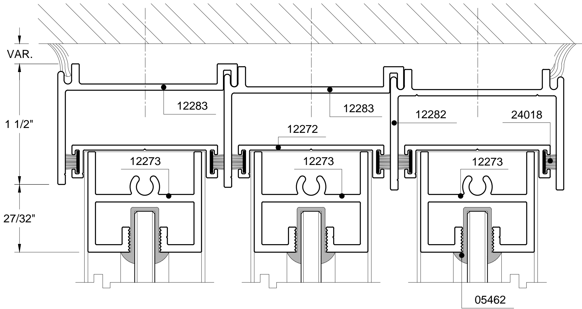
50 DOOR HEAD
